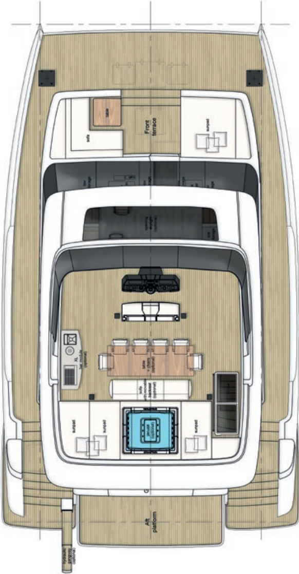
FLYBRIDGE
